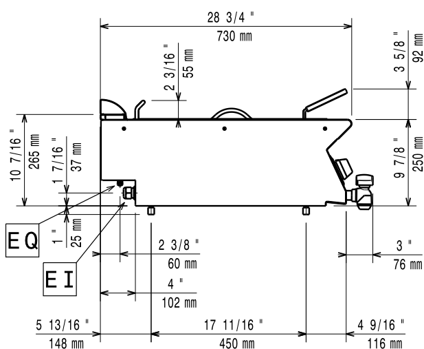
Oldalnézet
